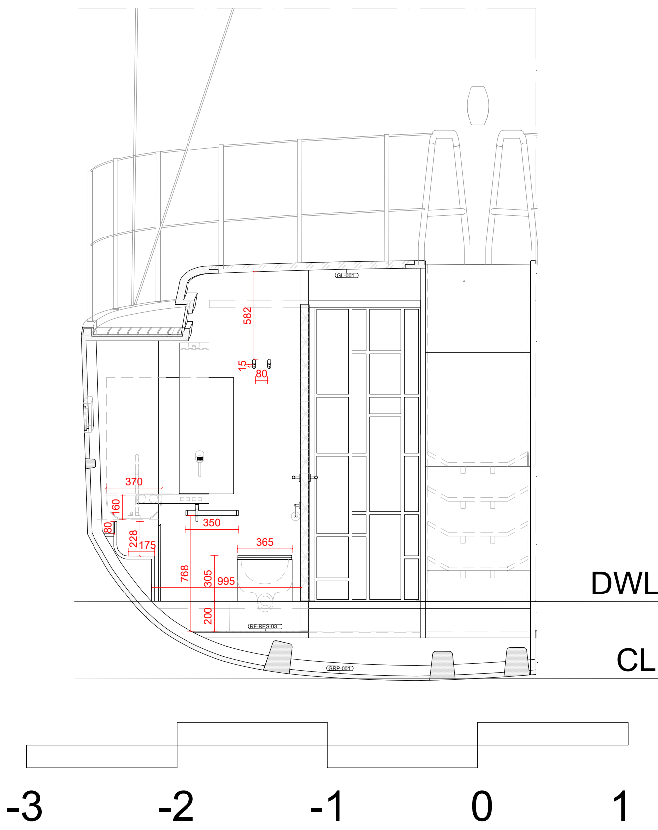
SEZIONE TRASVERSALE DD' | PRORAVIA
