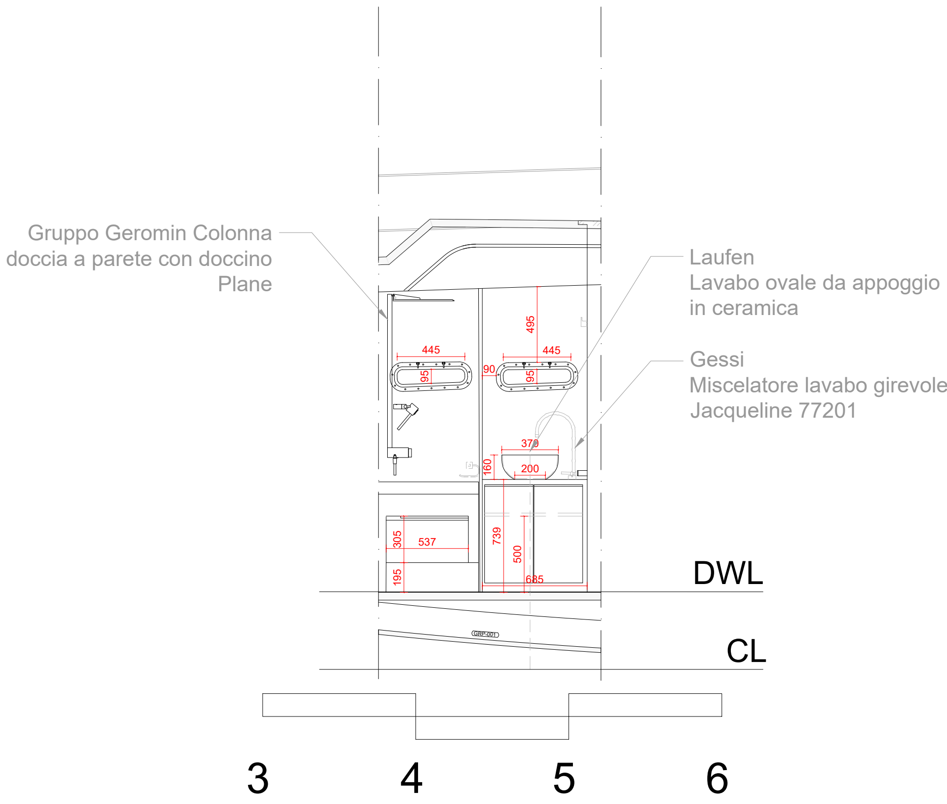
SEZIONE LONGITUDINALE AA
