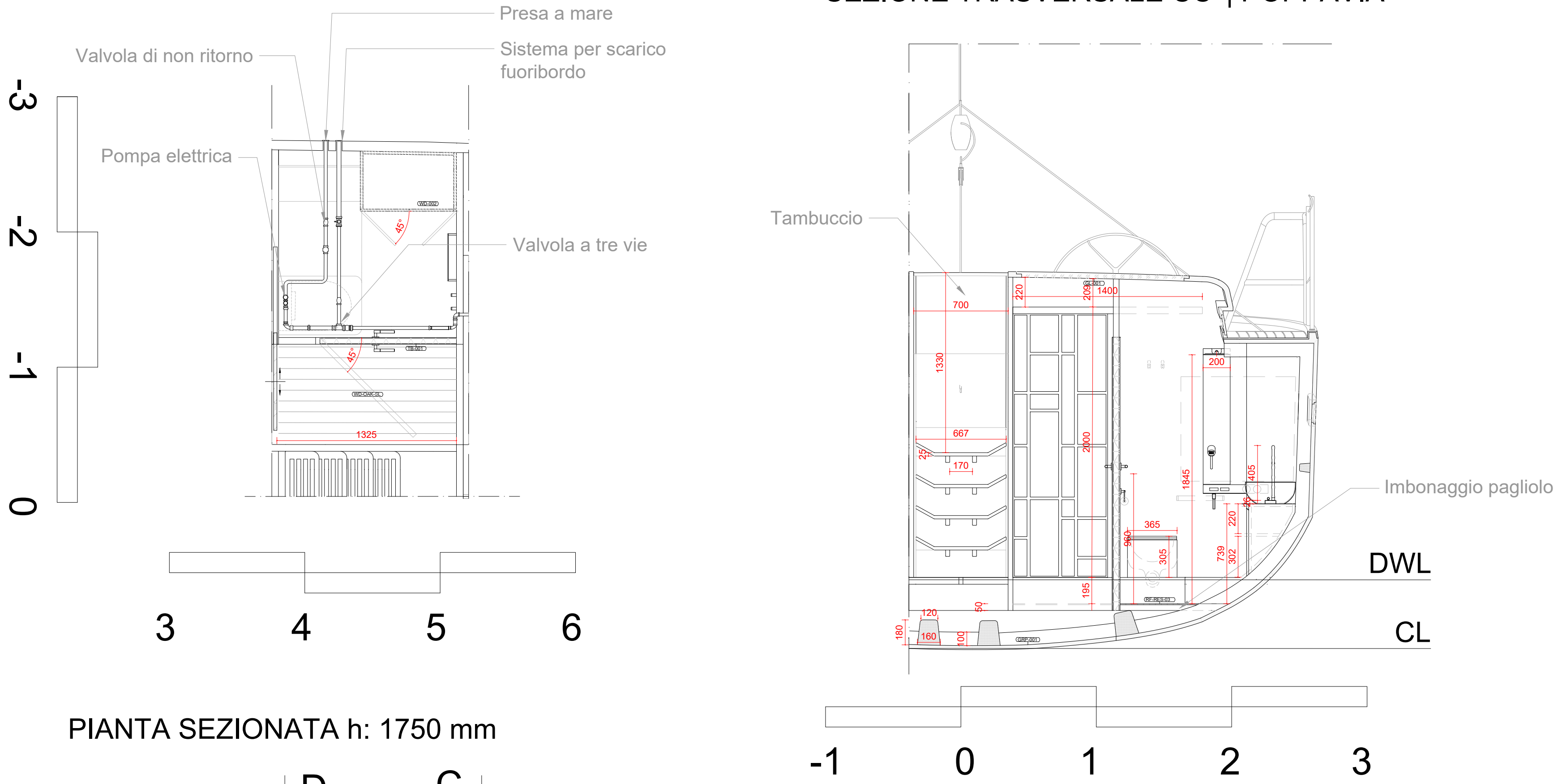
SEZIONE TRASVERSALE CC' | POPPAVIA
