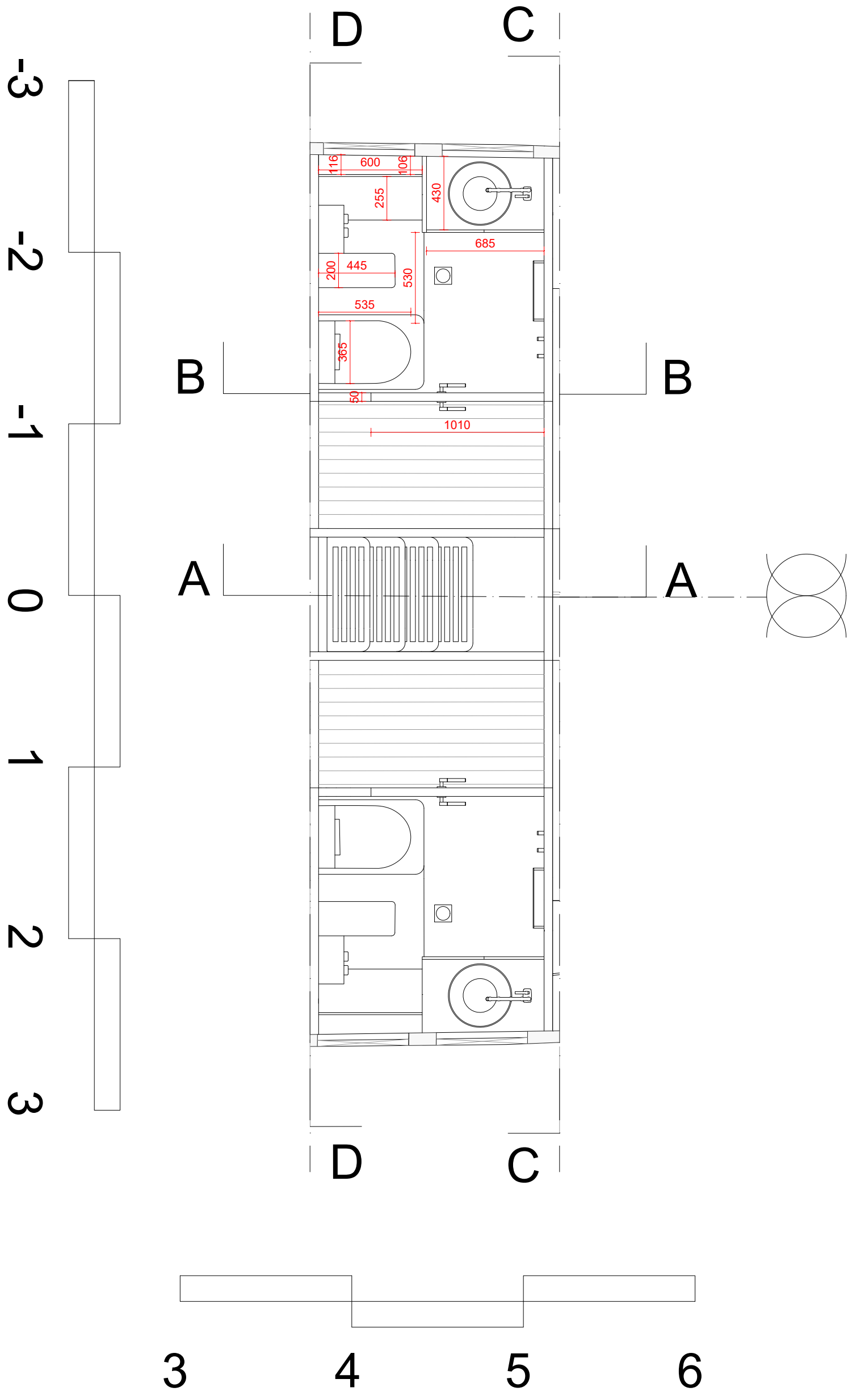
PIANTA SEZIONATA h: 1750 mm
